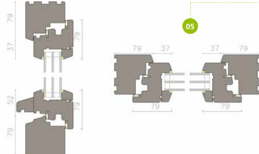
IV80 mit Wasserschenkel
