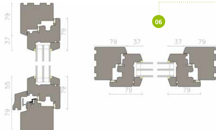
IV80 mit vorgehängen Wasserschenkel
