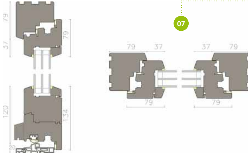
IV80 Terrassentür mit flacher Schwelle (Transit)
