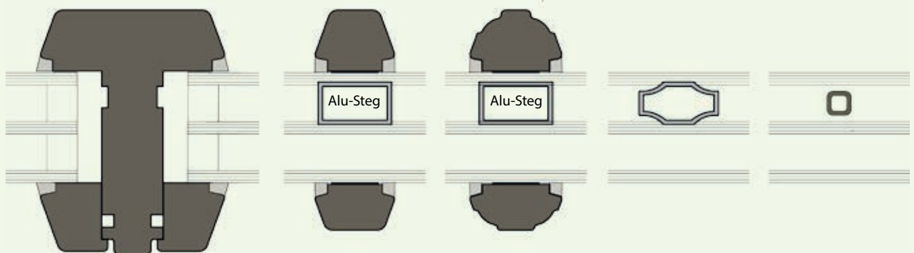
Glasteilende Holzspresse
